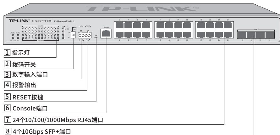
图1-1 TL-SH6428工业级前面板示意图
