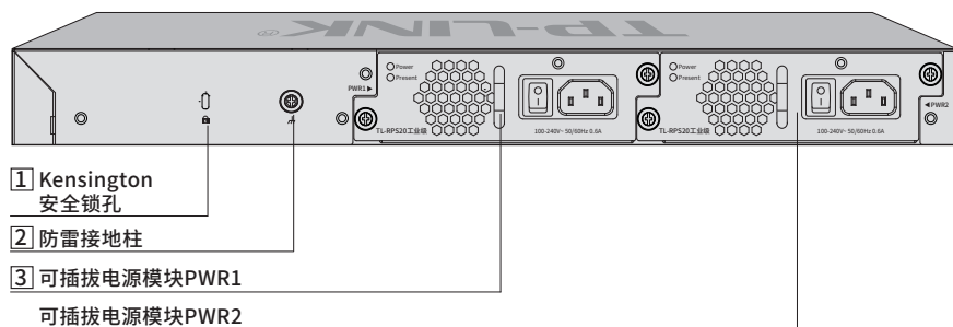
图1-2 TL-SH6428工业级后面板示意图
